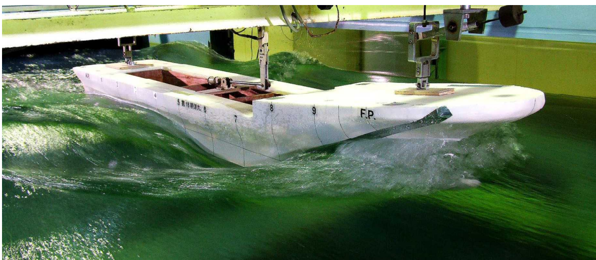
— 第18明洋丸 ( F_n = 0.388 ) —
