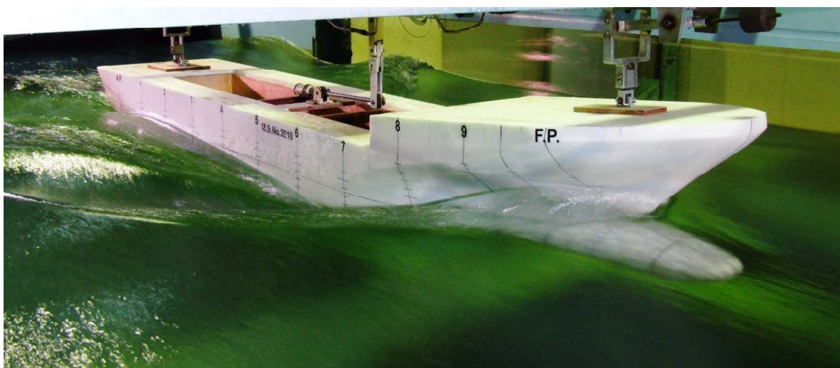
— M改I船型 ( F_n = 0.371 ) —
